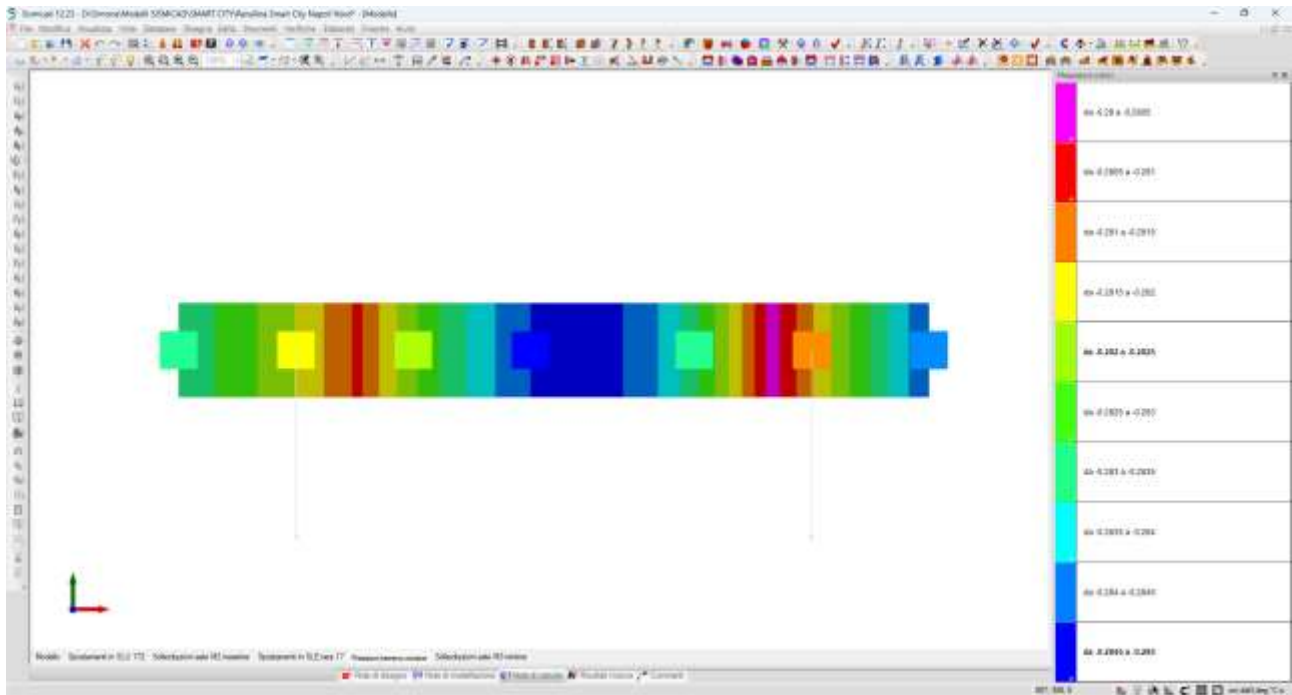
Figura 2. Pressioni massime in fondazione Fermata bus
